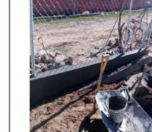
SOBRECIMIENTO
